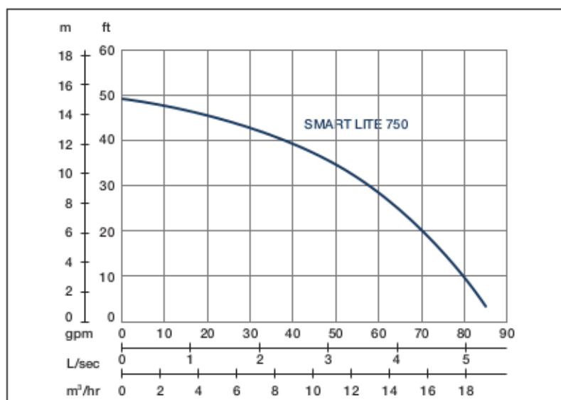
Charakterystyka pracy pompy SMART LITE 750
